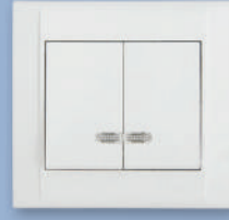
42001023 IŞIKLI KOMÜTATÖR TWO WAY SWITCH ILLUMINATED Gerilim / Rated Voltage 250V Akım / Rated Current 10A Koruma Derecesi / Protection IP20
